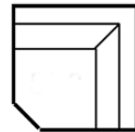
Modular Square Corner Unit W: 118cm D: 118cm H: 77-96cm SH: 47cm
